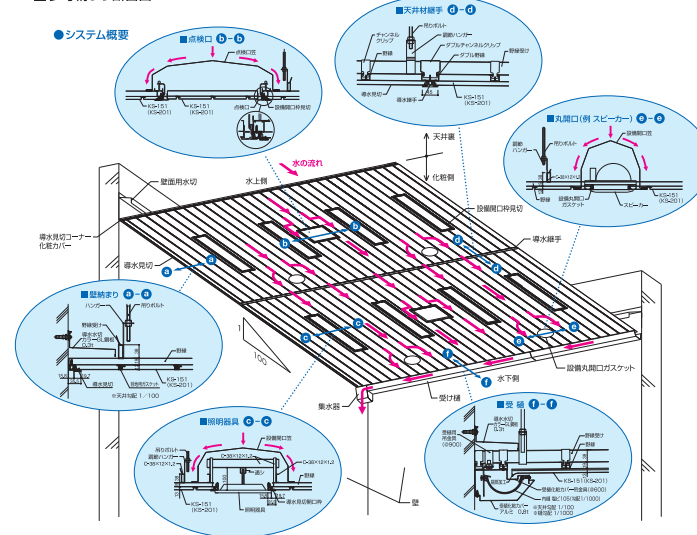
■参考納まり断面図
